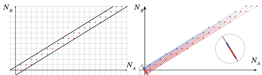
Рис. 4. Количество букв А и В среди первых n букв слова Фибоначчи
