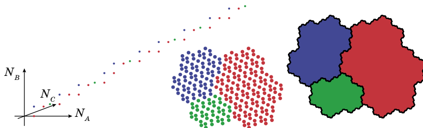
Рис. 5. Количество букв А , В и С среди первых n букв слова Трибоначчи и появление фрактала Розы
