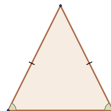
Рис. 11. Равнобедренный треугольник
